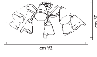
art. 5200/PL5 5 x max 60w E14 CE IP20
