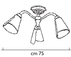
art. 5200/PL3 3 x max 60w E14 CE IP20
