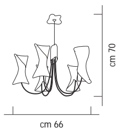
art. 6800/5 5 x max 60w G9 CE
