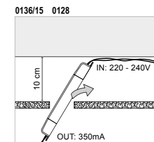
Installazione senza cassaforme Installation without wall box
