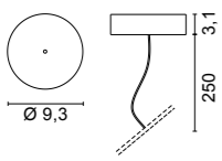
0946 Rosone completo di cavo di alimentazione. Ceiling rose with cable. .01 Bianco - White
