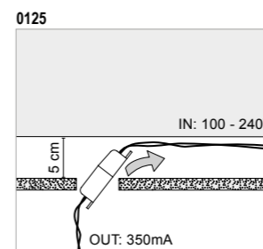
Installazione senza cassaforme Installation without wall box
